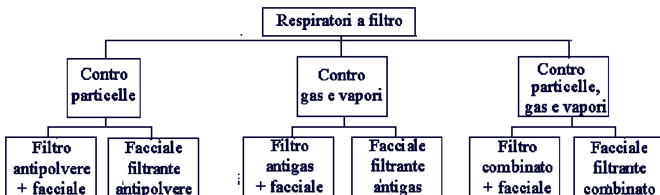
figura 3 Classificazione dei respiratori a filtro
