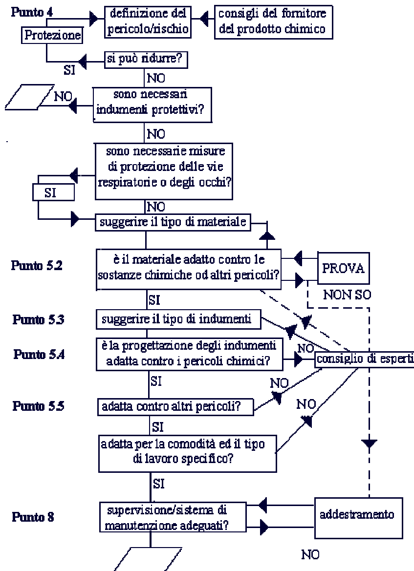
Fig. 1 - Procedura di selezione - Diagramma di flusso
