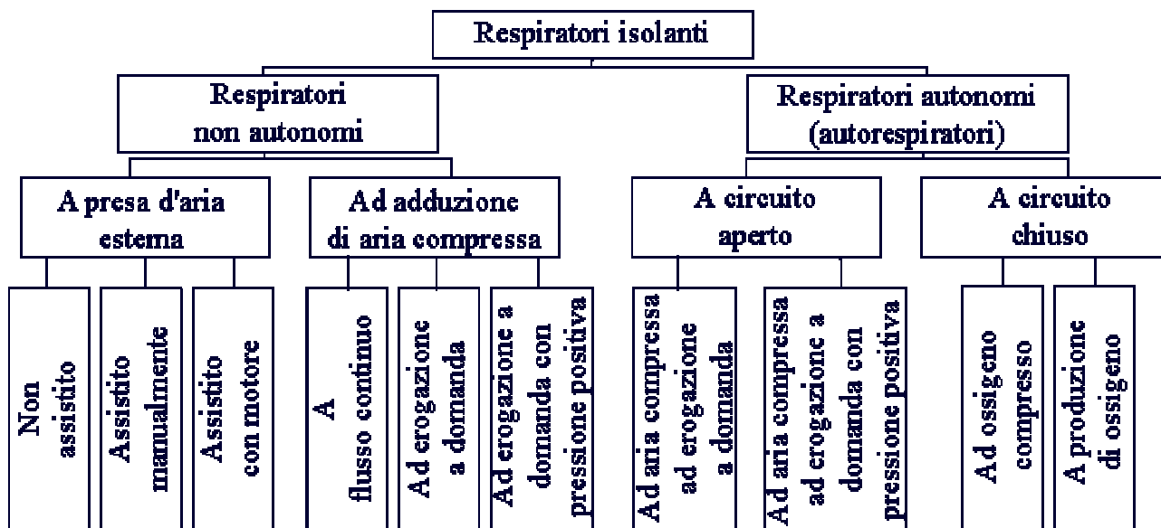
figura 10 Classificazione dei respiratori isolanti
