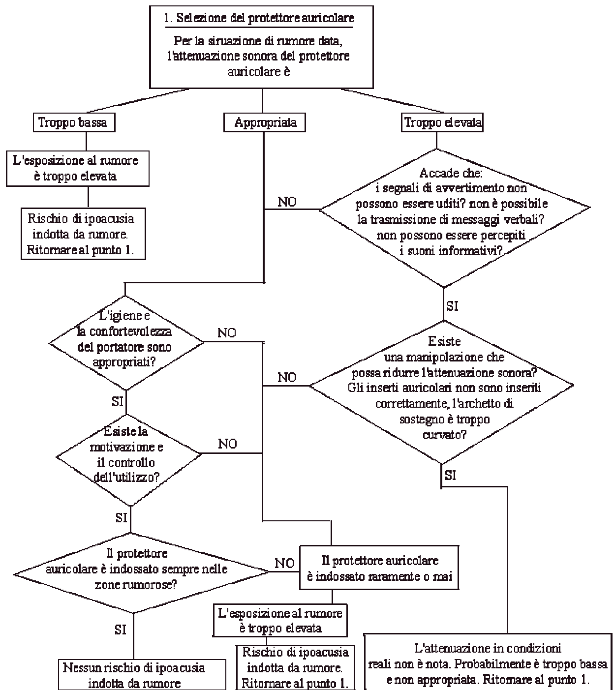
Fig. 3 - Fattori da tenere in considerazione per la selezione dei protettori auricolari
