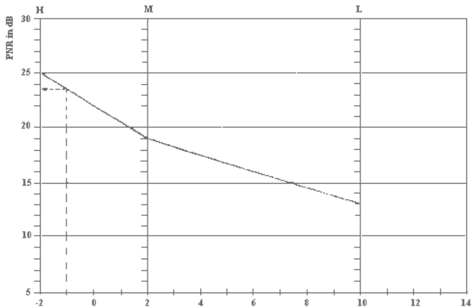
Fig. A 1 - Grafico che consente di ottenere il valore PNR senza effettuare calcoli
