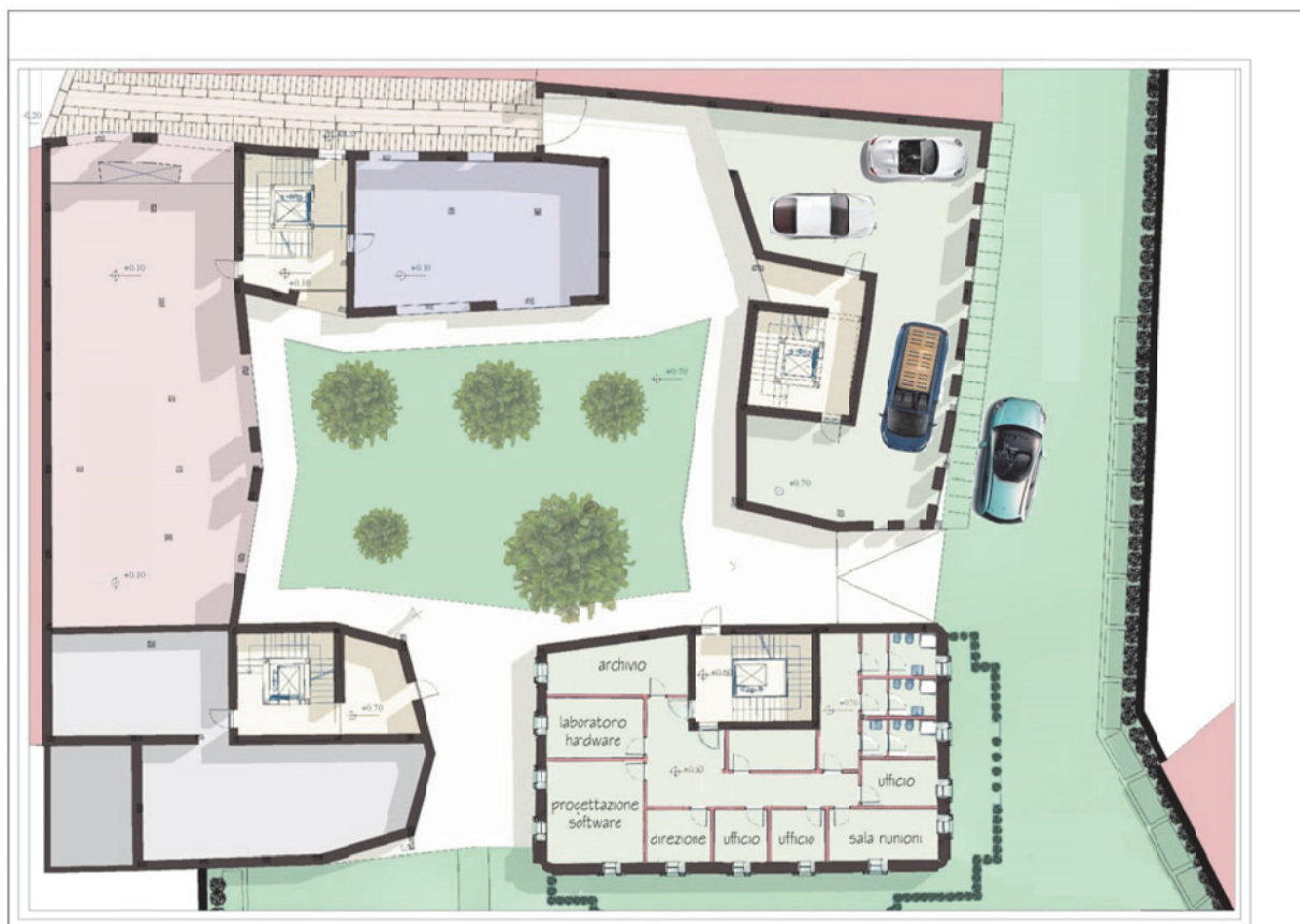
Planimetria degli uffici con inserimento nel comprensorio
