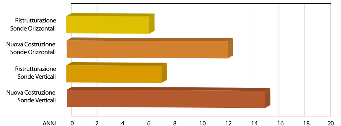
RISULTATI DELL'ANALISI IN TERMINI DI TEMPO DI RITORNO DELL'INVESTIMENTO (NON ATTUALIZZATO) PER UN'ABITAZIONE MONOFAMILIARE DI 100 - 120 \text{ M}^2 E POMPA DI CALORE DA 8 \text{ KW}_t
