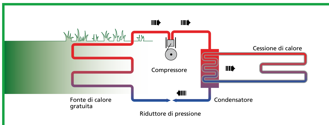
SCHEMA DI FUNZIONAMENTO DI UNA POMPA DI CALORE GEOTERMICA IN FASE DI RISCALDAMENTO
