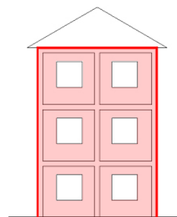
Fig. 1 – Regola per il calcolo della trasmittanza termica corretta dei componenti opachi rivolti verso l'esterno.
