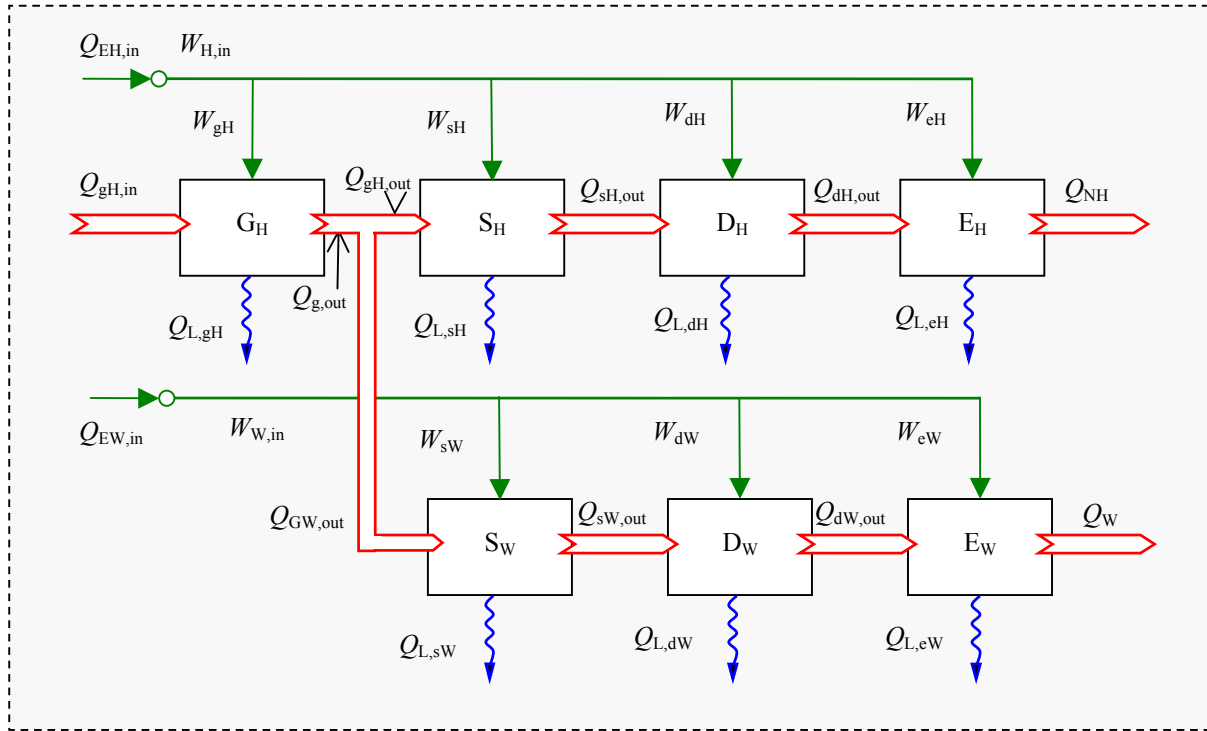
Figura 7 – Schema di calcolo dell'energia primaria per impianti combinati per la climatizzazione invernale e la produzione di acqua calda sanitaria (Fonte: prEN 15316)
