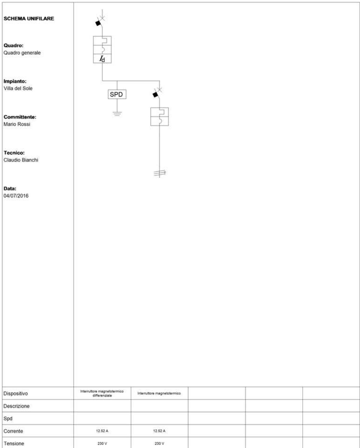
Fig. 6: Schema unifilare quadro "Quadro generale"
