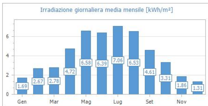
Fig. 1: Irradiazione giornaliera media mensile sul piano orizzontale [kWh/m 2 ]- Fonte dati: UNI 10349:2016 - Stazione di rilevazione: Mirabella Eclano
